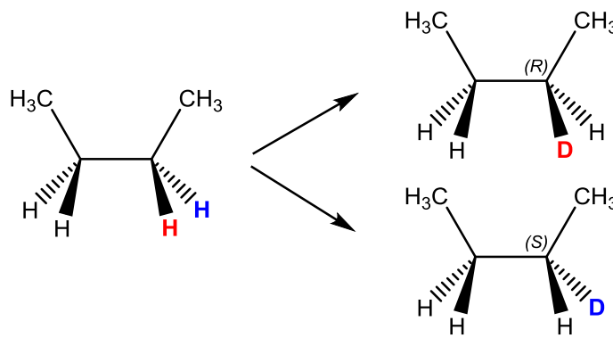
Enantiotope Protonen
