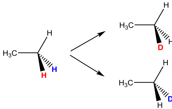
Homotope Protonen
