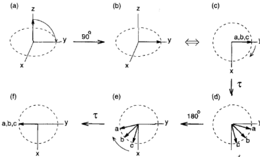
Messung der Spin-Spin-Relaxationszeit T_2 mit dem Spin-Echo-Experiment .
