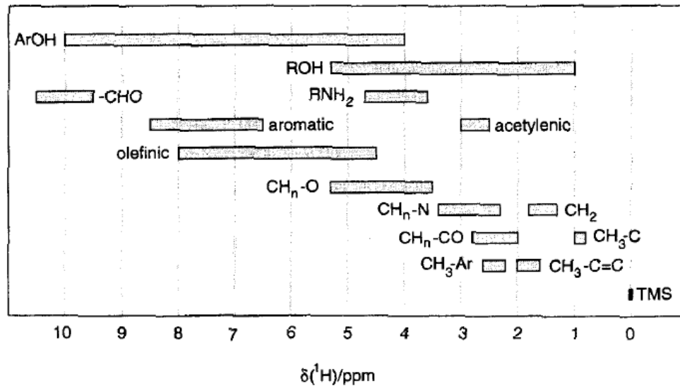
Charakteristische Bereiche für die ^1\text{H} -chemische Verschiebung einiger funktioneller Gruppen
