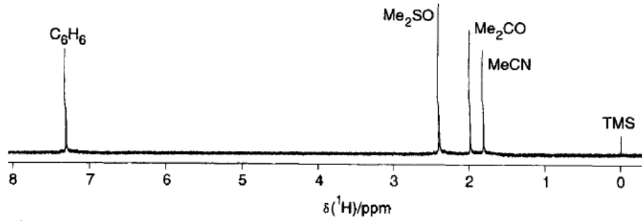
^1\text{H-NMR} -Spektrum (400 MHz) eines Lösungsmittelgemisches
