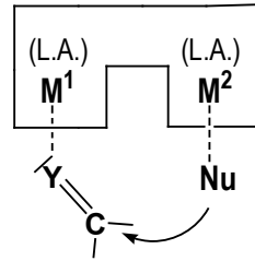
Doppelte Lewis-Säure-Aktivierung, Nu = Reaktand, CY = Substrat
