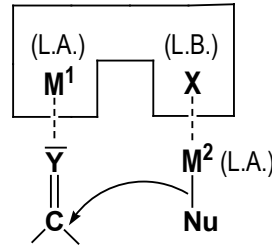
Lewis-Basen- und doppelte Lewis-Säure-Aktivierung
